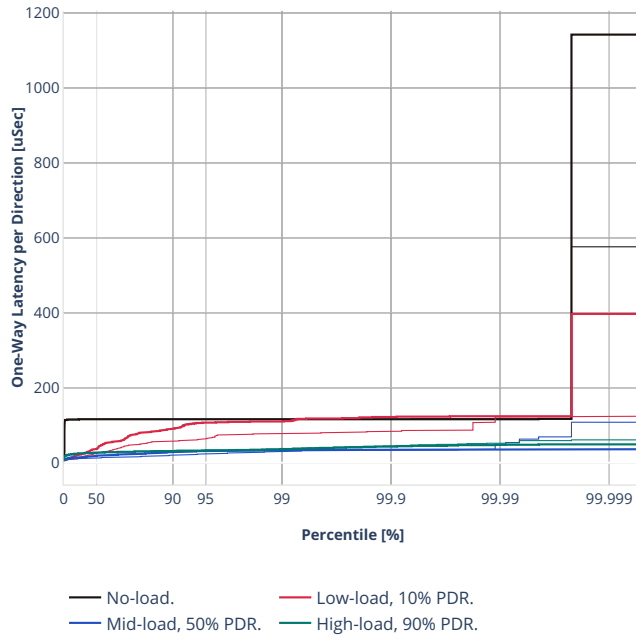
Latency: rdma-ethip4-ip4scale20k
