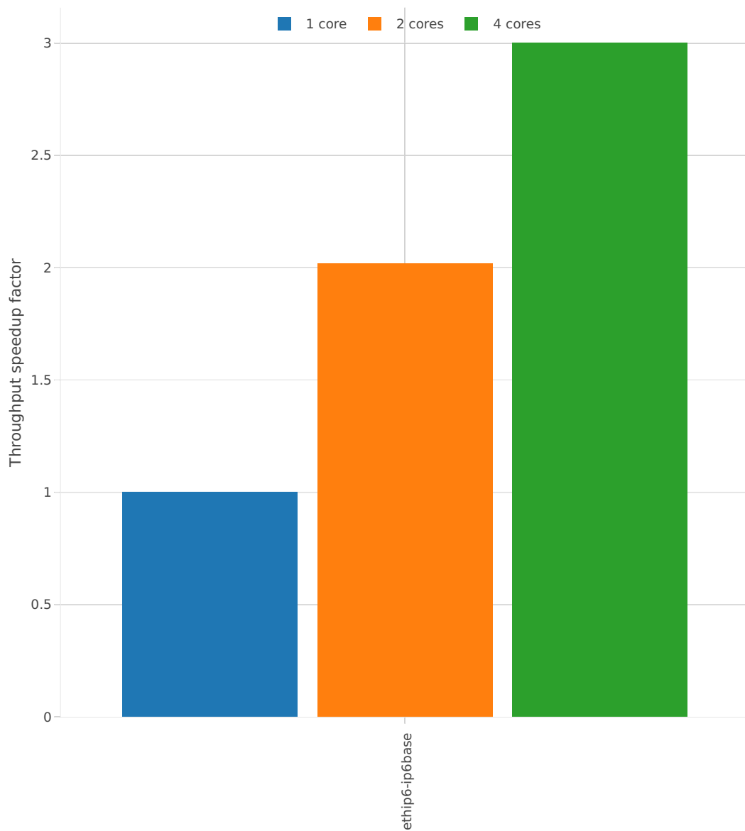
78B-*-ethip6-ip6(base|scale)*ndrdisc
